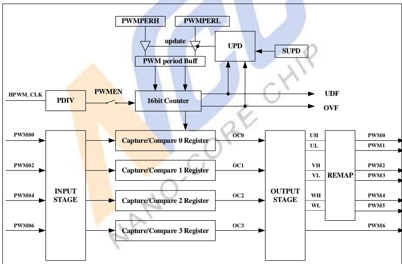
图 21-1 PWM设计框图
