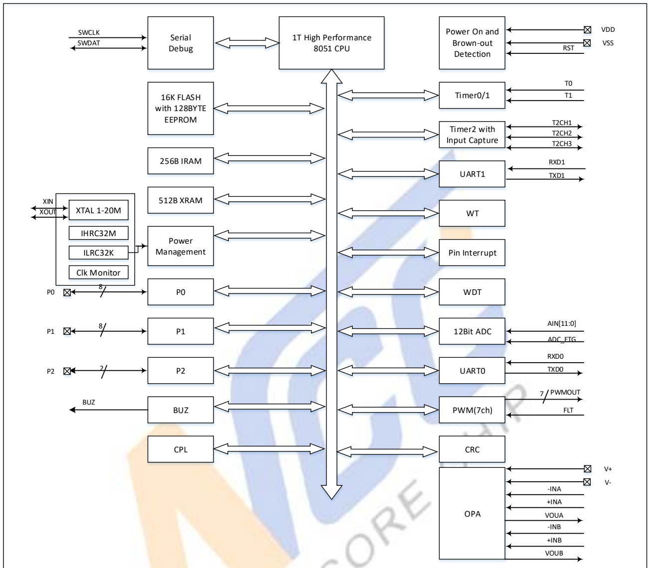
图 3-1 设计框图
