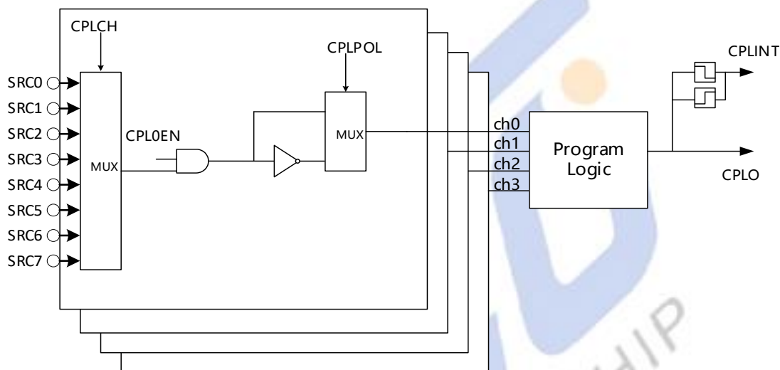
图 17-1 CPL 内部框图
