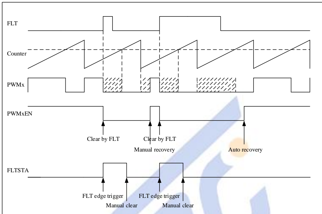
图 21-14 硬故障保护
