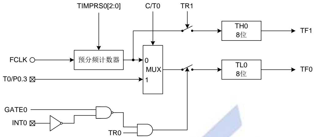
图 13-4 定时器 0 工作模式 0
