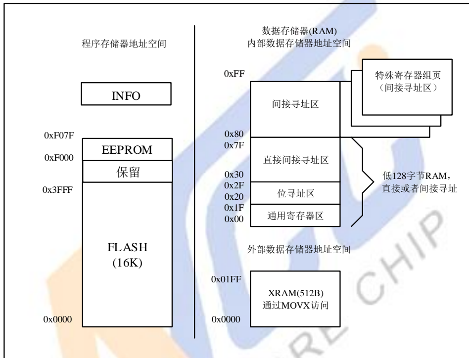
图 6-1 ATM8F7040 存储器空间
