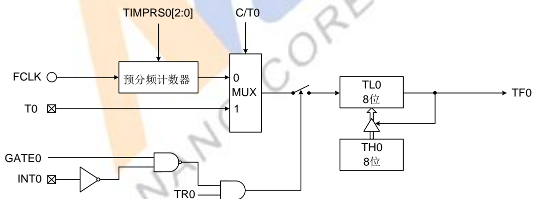
图 13-3 定时器 0 工作模式 0
