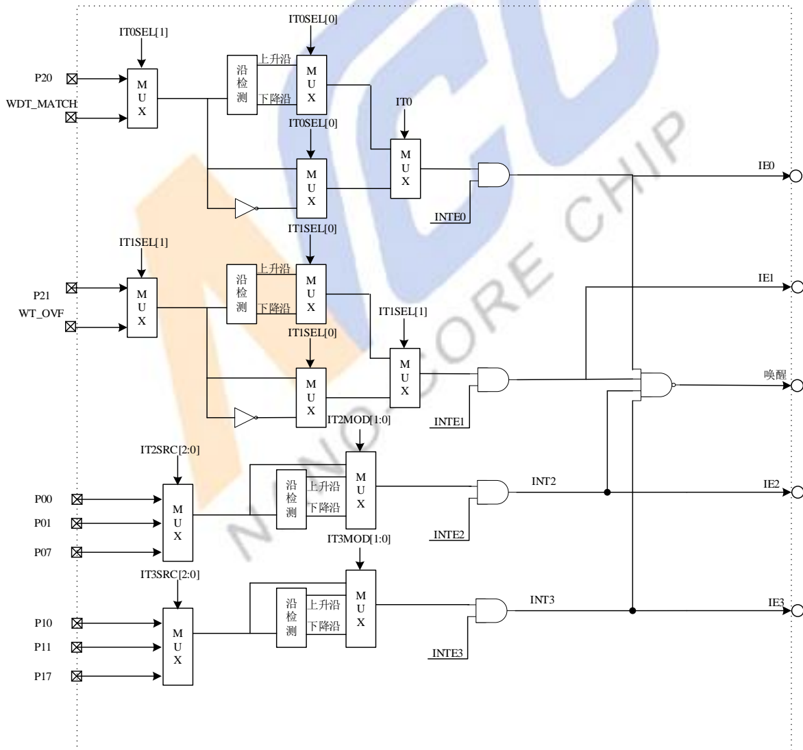
图 9-1 中断结构图
