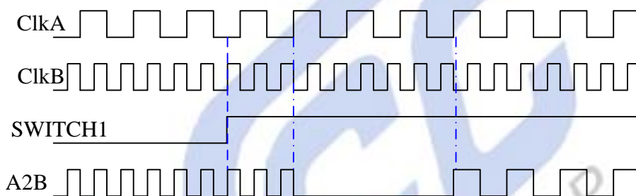
图 11-2 快速时钟切换到慢速时钟
