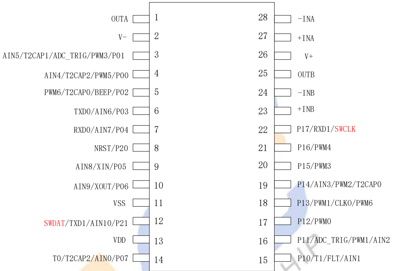
图 4-1 TSSOP28 引脚图
