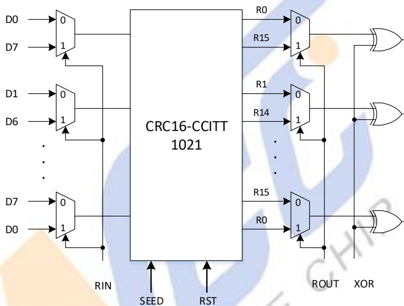
图 16-1 CRC 结构图
