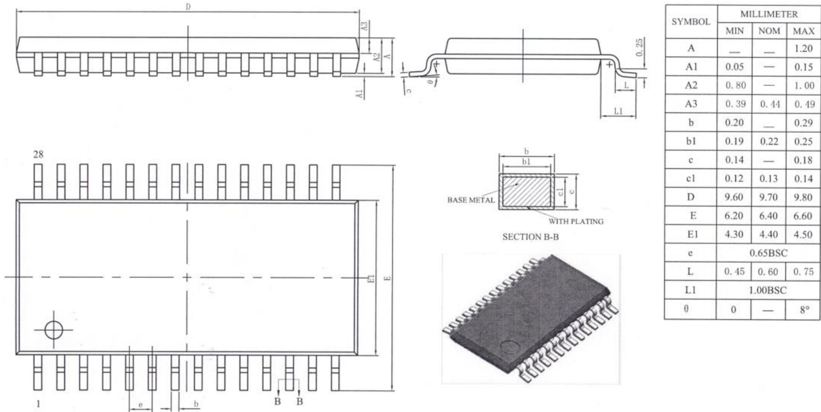
图 26-1 TSSOP28 封装尺寸图
