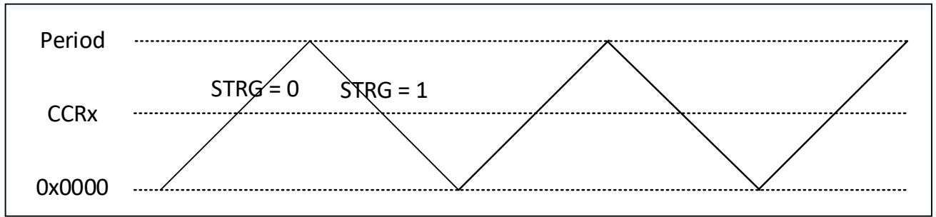
图 21-3 连续中央对齐示意图
