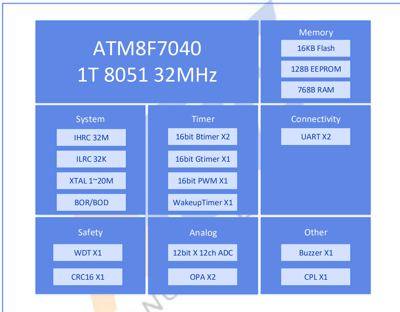
图 1-1 功能组成框图
