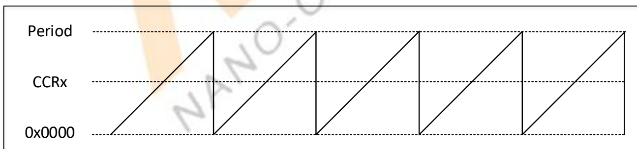
图 21-2 连续边沿对齐示意图
